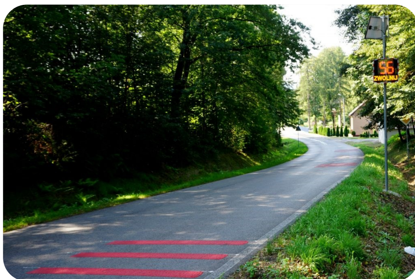
Widok na jezdnię, czerwone oznakowanie poziome drogi i tablicę solarną do pomiaru prędkości
